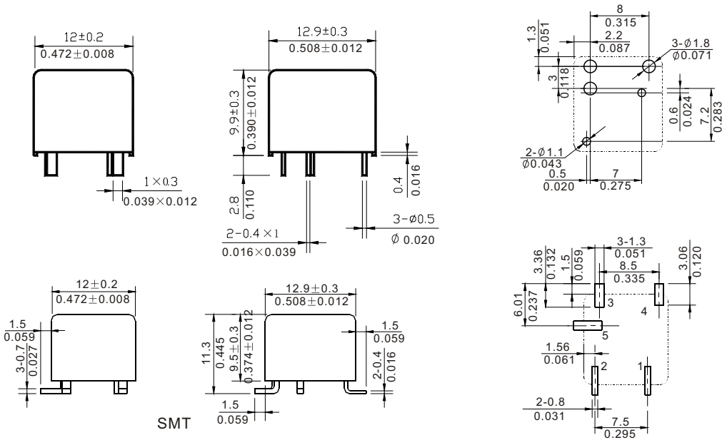
Dimensions
